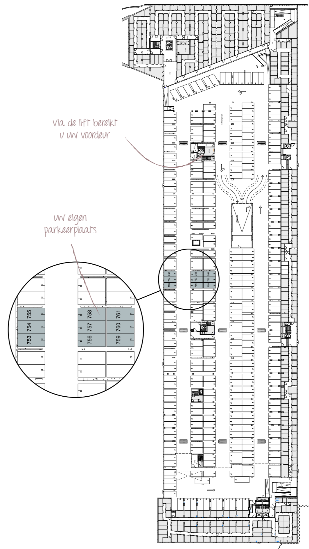
Parkeerlaag en bergingen, laag -1
